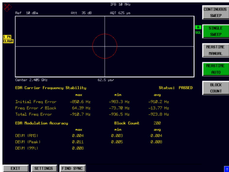
Bild 3-12 Trägerfrequenzstabilitäts- und Modulationsgenauigkeitsmessung (EDR)
