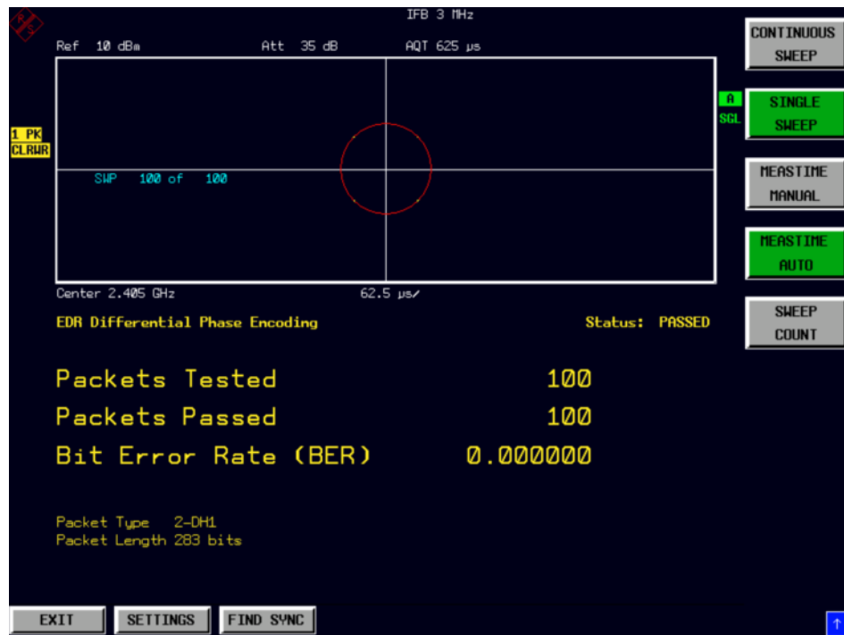
Bild 3-13 Differential Phase Encoding-Messung (EDR)
