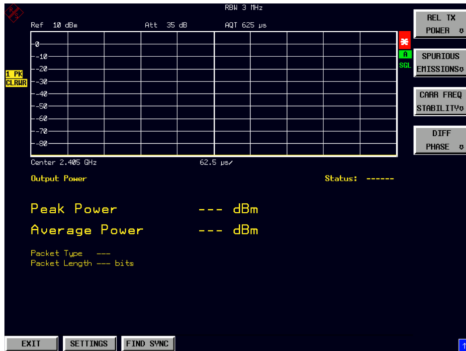
Bild 3-8 Enhanced Data Rate-Messungen (EDR)
