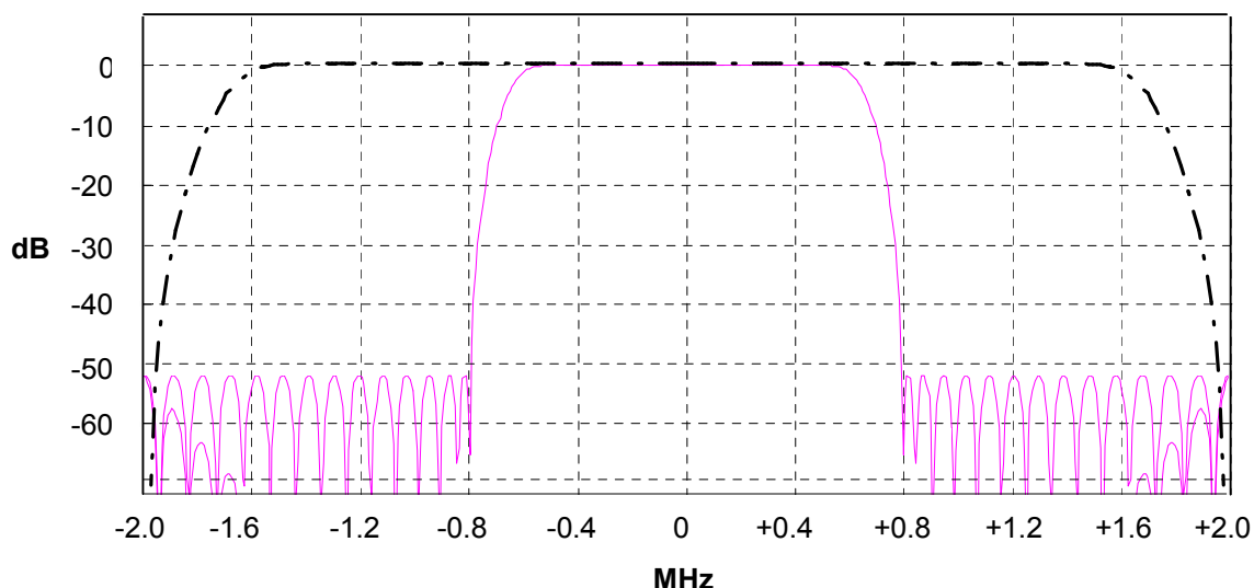
Bild 1-2 Selektion der Digitalfilter Strichpunktierte Kurve: Standardfilter bei 4 Points / Symbol Durchgezogene Kurve: Zuschaltbares Filter, fix für alle Points / Symbol Einstellungen
