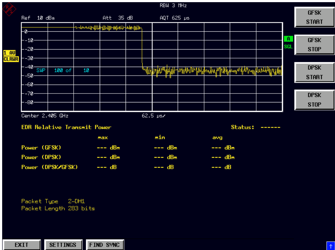
Bild 3-10 Untermenü mit den Einstellungen für die Berechnung der mittleren Leistung (Average Power)
