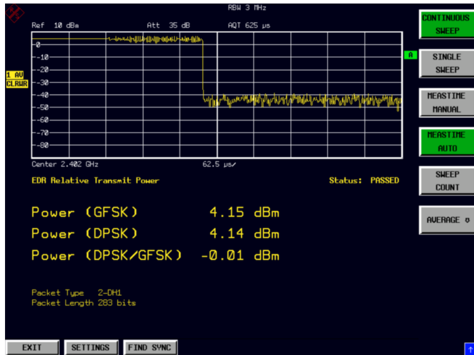
Bild 3-9 Messung der relativen Übertragungsleistung (EDR)
